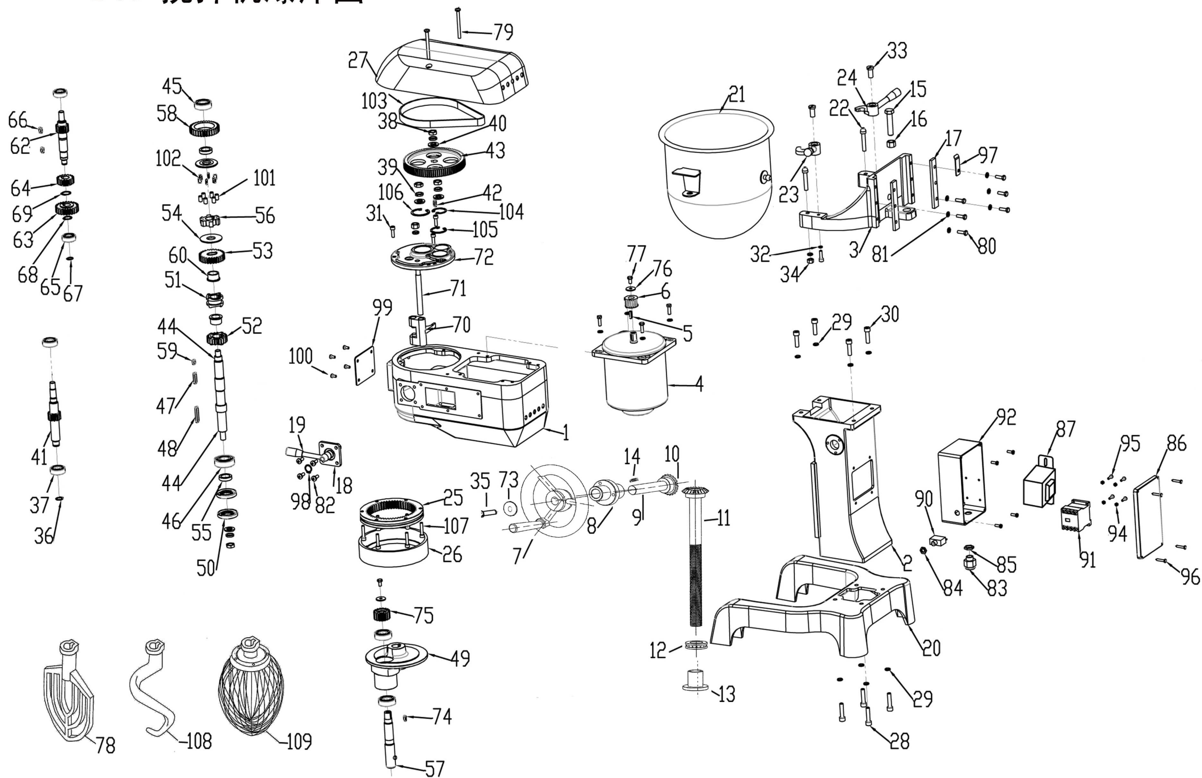
B40 搅拌机爆炸图
